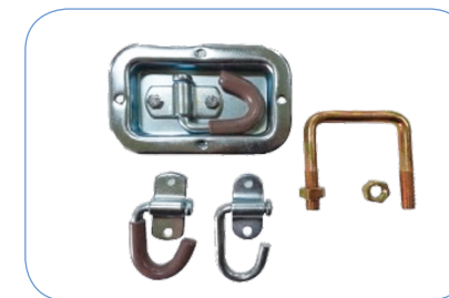
J바고리 (회전식 / 측면식), U형 바고리 J Bar rings (Rotary / Side type), U-type bar ring J바프ック(回転式 / 側面式), U字フック
