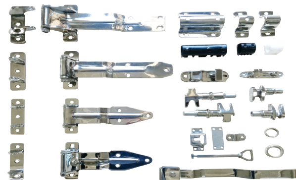
비바+부싱 / 티바 / 티고리 BB+Bushing / T Bar / T-Ring BB+ブッシュ / Tバー / T掛け
