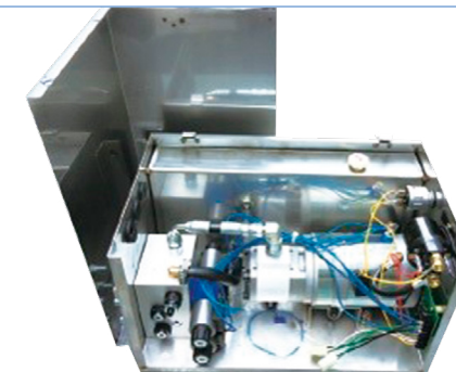
유압 UNIT (12V, 24V) Hydraulic UNIT (12V, 24V) 油圧ユニット (12V, 24V)
